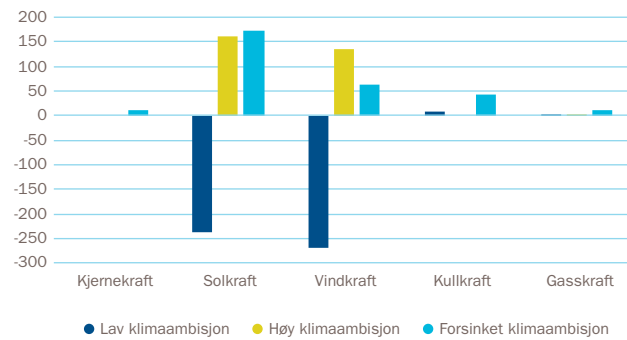
27 Endringer i utbygd kapasitet (GW) i kraftsektoren i Europa for ulike klimaambisjoner i forhold til Lavutslippsscenarioet
