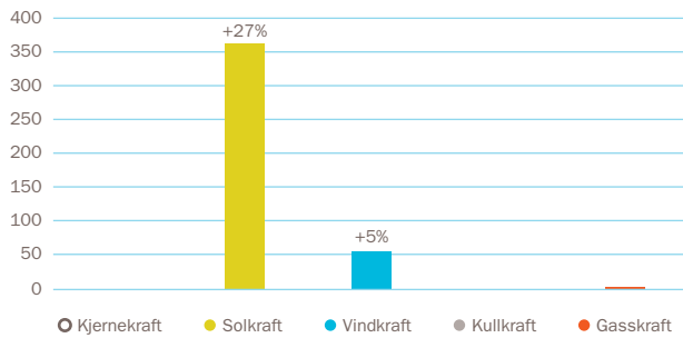
34 Endringer i kraftkapasitet (GW) fra Lavutslippsscenarioet i 2050 når direkte elektrifisering begrenses.
