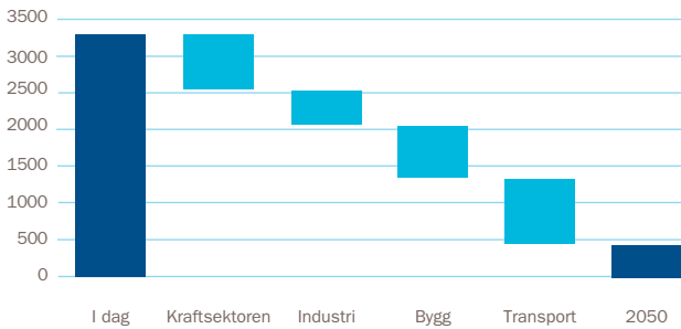
28 Utslippsreduksjoner i Europa i Lavutslippsscenarioet fra i dag til 2050 per sektor (energi relaterte CO 2 -utslipp i Mt).
