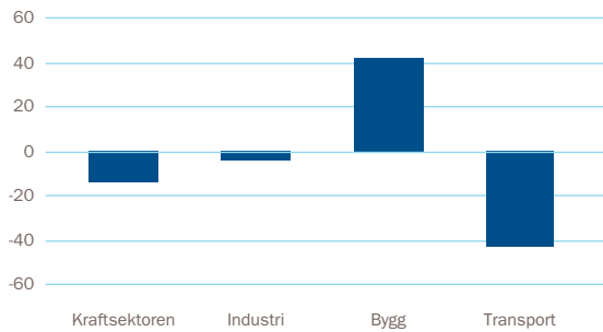
33 Endringer i utslipp per sektor i 2050 med lavere elektrifisering (Mt CO 2 )
