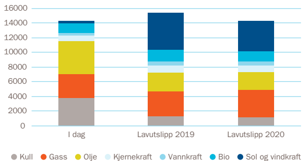
4 Global etterspørsel etter primærenergi i dag og i 2050 i Lavutslippsscenarioet (Mtoe).
