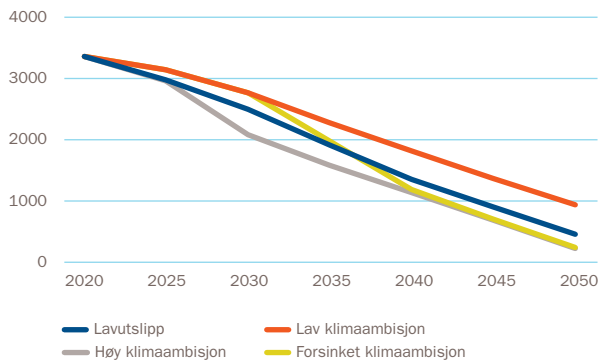
26 Utslippsbaner i Europa med ulike klimaambisjoner (energirelatert CO 2 -utslipp i Mt).
