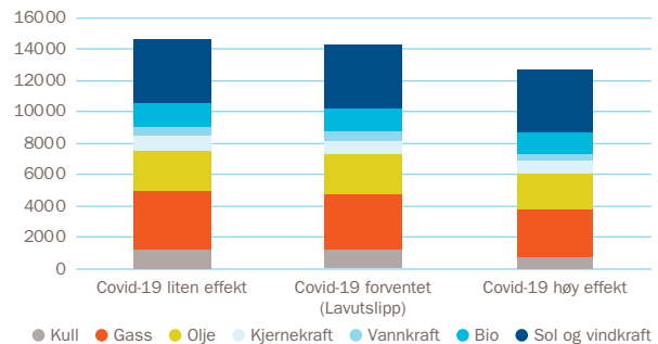
5 Global etterspørsel etter primærenergi i 2050 ved ulike langtidseffekter av Covid-19-pandemien (Mtoe).
